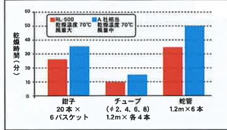
3種類の乾燥物を同時に乾燥させたときの乾燥時間
