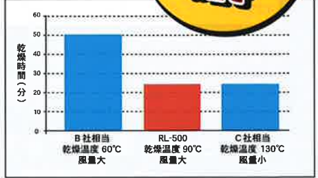
鉛子 60本 × 6バスケットの乾燥時間
