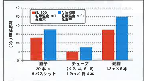
3種類の乾燥物を同時に乾燥させたときの乾燥時間
