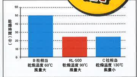
銅子 60本 × 6バスケットの乾燥時間
